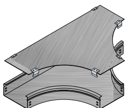
TEE HORIZONTAL HORIZONTAL TEE
