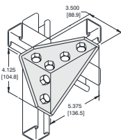
UL-1957 Conector de esquina reforzado izquierdo 6 orificios Six hole (left hand) gusseted corner connection
