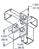
UL-1034 Conector "T" angular 90° izquierdo 4 orificios Four hole (left hand) offset bent teeangle
